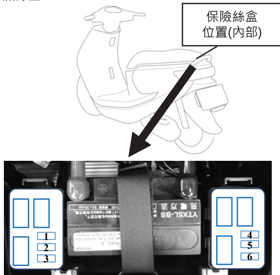
保險絲盒 1
